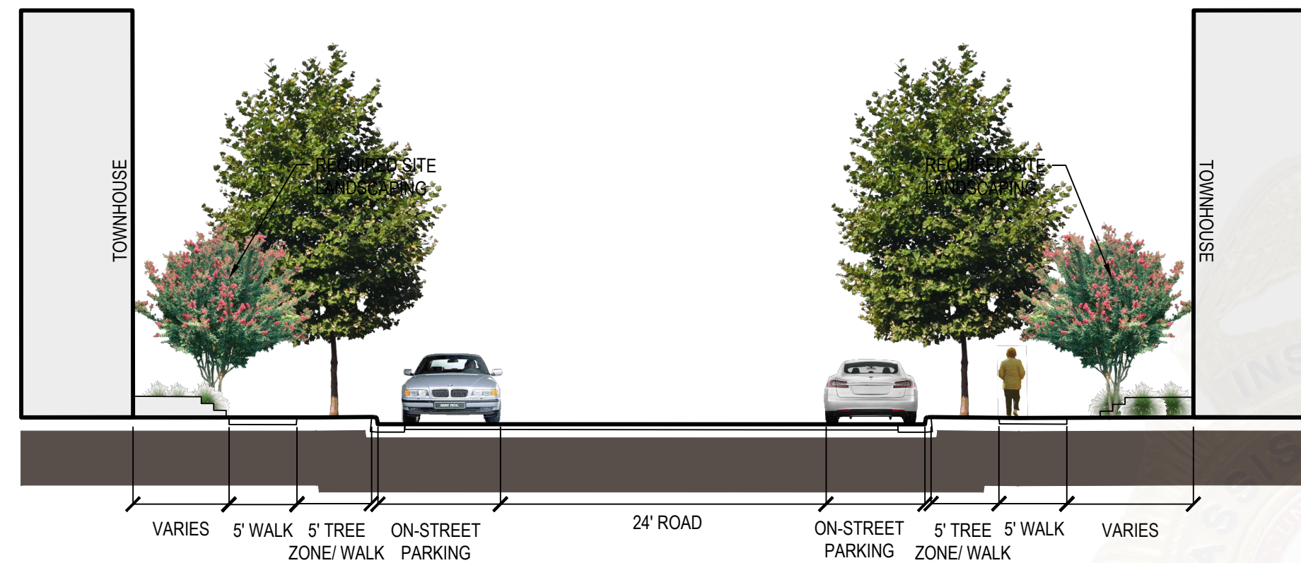
8 ROAD 'B' Scale: 1" = 10'
